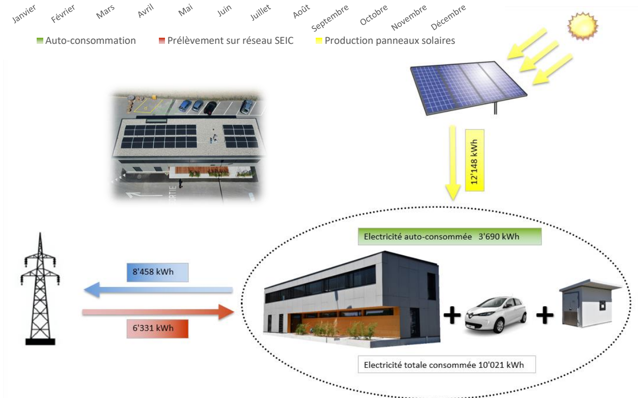
Fig. 12 – Schéma de la production et de la consommation annuelles d'électricité en 2019
